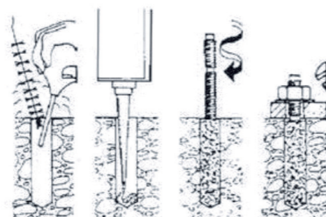
Forer - Nettoyer - Injecter la résine Introduire l'élément à sceller en tournant
